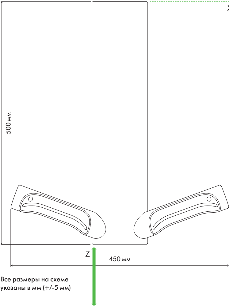
Вид спереди
