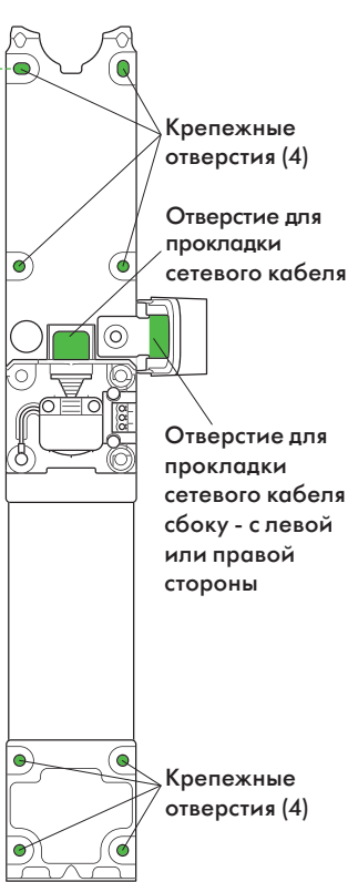
Задняя стенка
