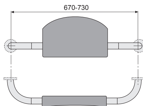
HEWI Serie 801 Bestell-Nr. 801.51.900/801.51.910
