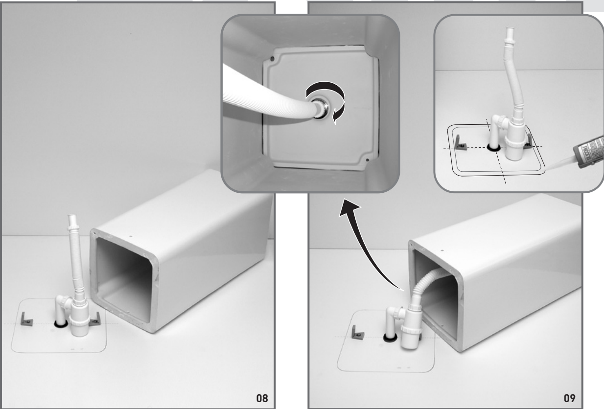
08 Allestimento per il fissaggio del lavabo: serrare bene le staffe nella posizione corretta. Preparation for the basin fixing: firmly fasten the brackets in the correct position.
