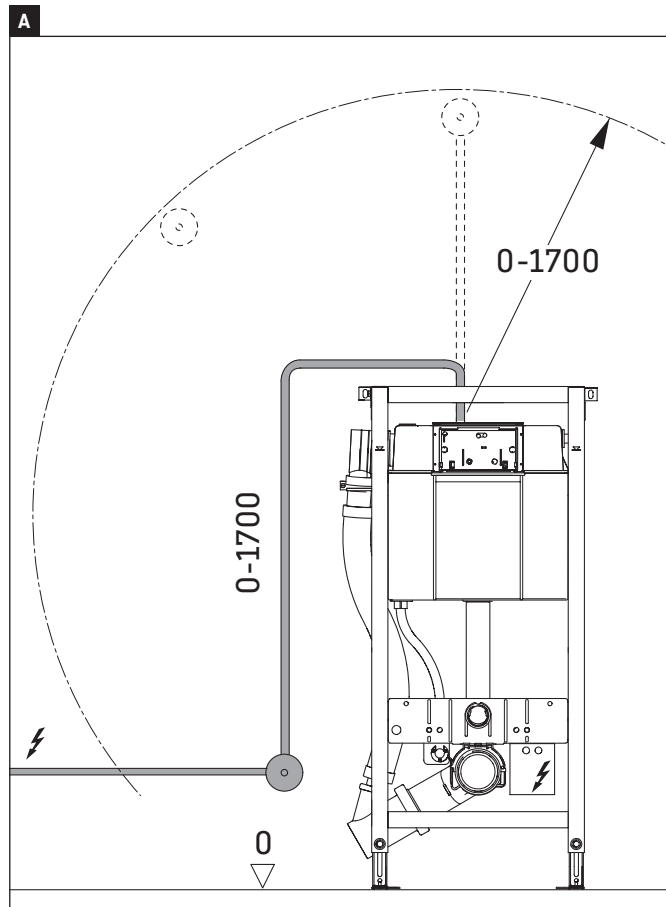
Ochranné zóny podľa DIN VDE 0100-701
